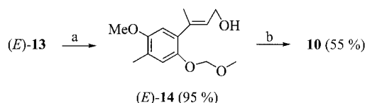
Scheme 3. a) DIBALH, THF, 0 °C. b) \text{OsO}_4 , NMO, t\text{BuOH} , \text{H}_2\text{O} , THF, 0 °C.
